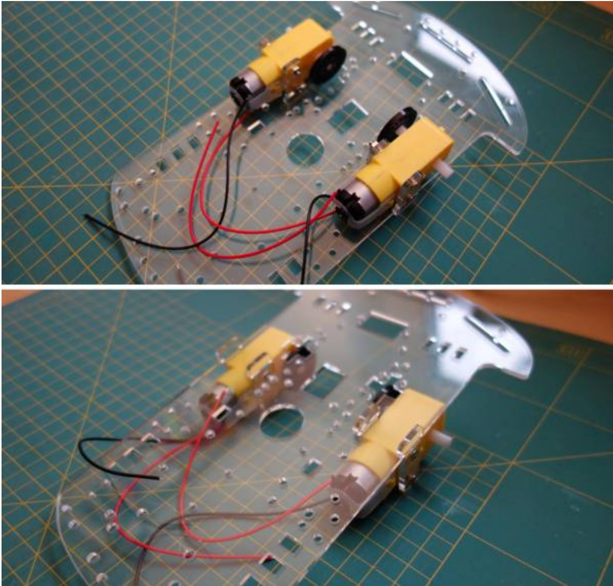
Schlepprad Vorbereitung:
